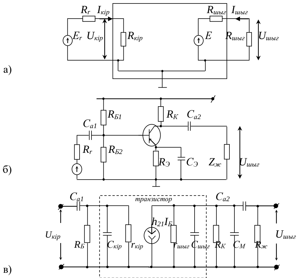
9-сурет. RC-күшейткіш каскадының схемасы
