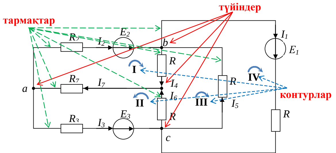
10-сурет. Электр тізбегінің мысалы
